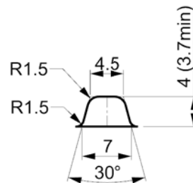
Dettaglio Tacca di Centraggio - Scala 2:1 Orientation Mark - Scale 2:1
