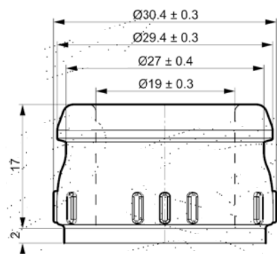
Dettaglio Imboccatura - Scala 2:1 Finish Detail - Scale 2:1
