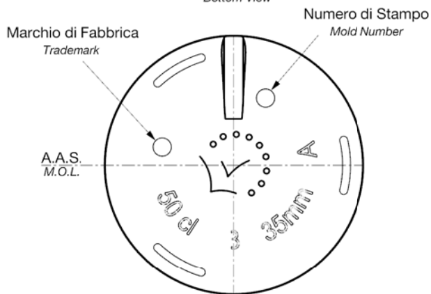
Vista dal Fondo Bottom View
